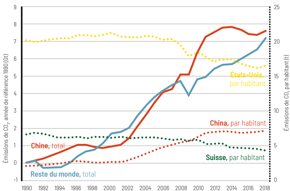
Figure 7 : Total des émissions de CO 2 (trait plein, axe de gauche) et émissions de CO 2 par habitant (trait en pointillé, axe de droite) en comparaison avec les États-Unis, la Suisse et le reste du monde (sources : Indicateurs du développement dans le monde, Banque mondiale ; Global Carbon Project).
